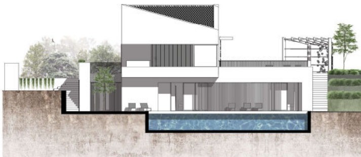
zapadno pročelje
